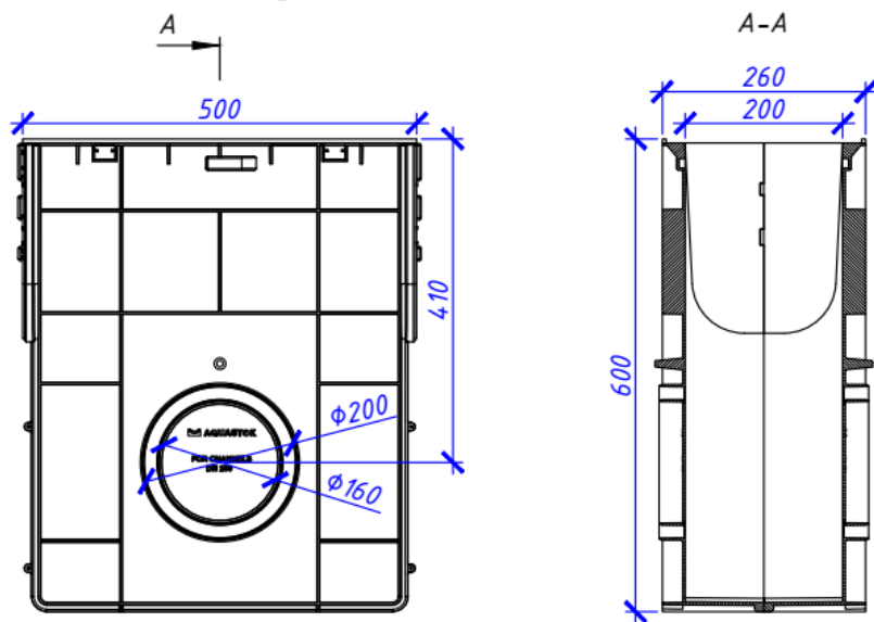
Пескоуловитель Норма Plastik DN200
