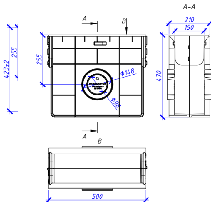
Пескоуловитель Norma Plastik DN150
