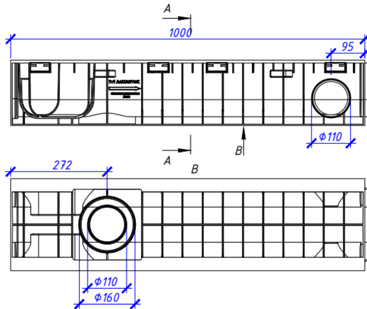
Лоток водоотводный Norma Plastik DN200 H280
