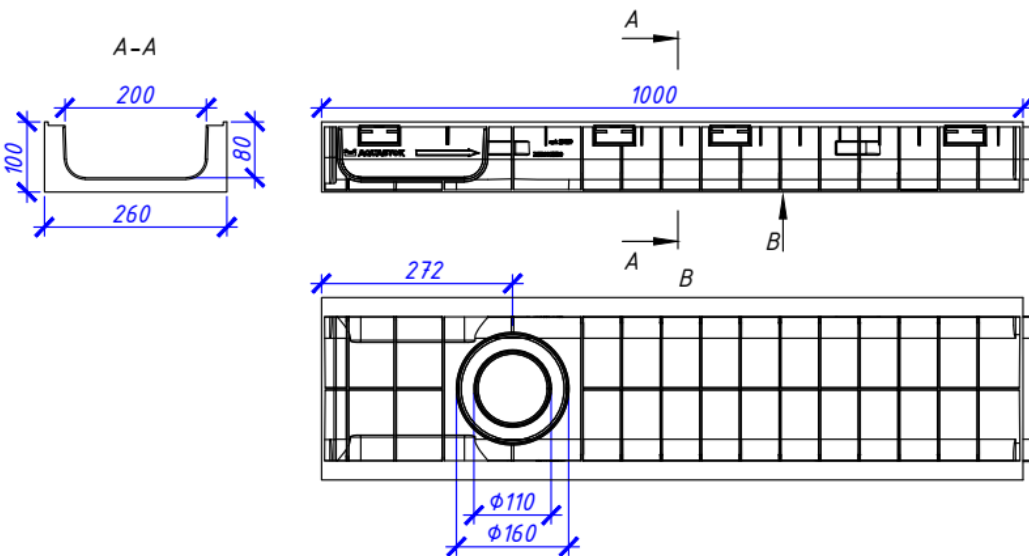
Лоток водоотводный Norma Plastik DN200 H100
