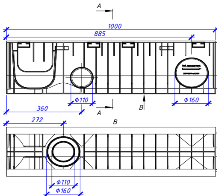
Лоток водоотводный Norma Plastik DN200 H280
