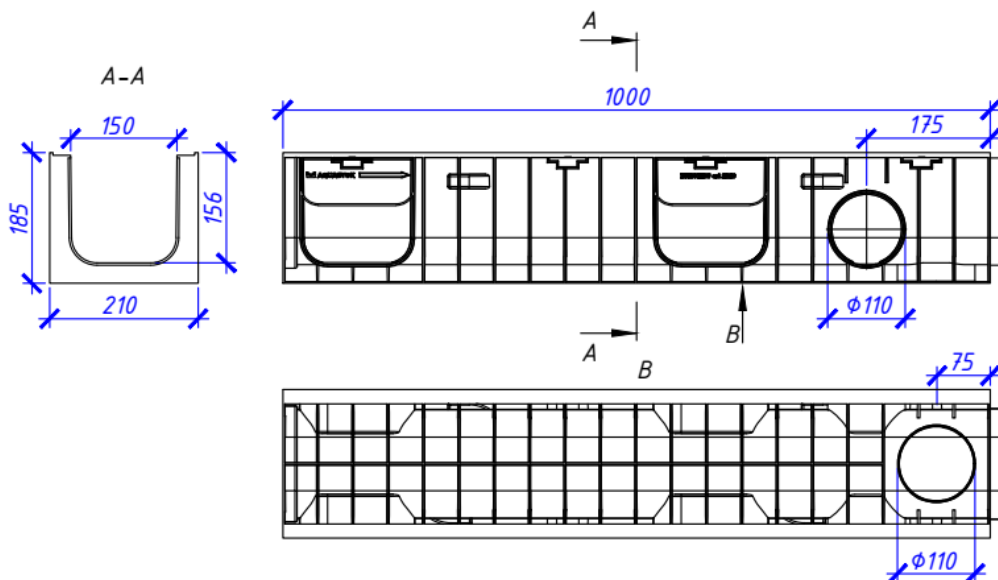
Лоток водоотводный Norma Plastik DN150 H185
