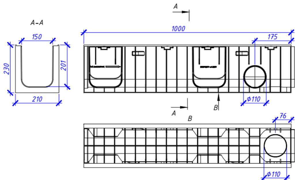
Лоток водоотводный Norma Plastik DN150 H230
