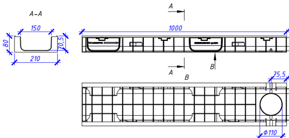
Лоток водоотводный Norma Plastik DN150 H80
